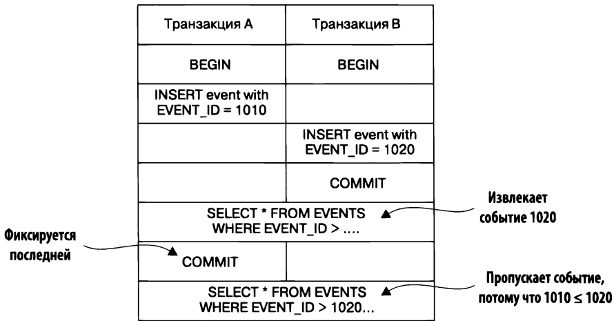
Рис. 6.6. Сценарий, в котором событие пропускается из-за того, что его транзакция А фиксируется после транзакции В. Опрашивающий запрос видит eventId=1020 и позже пропускает eventId=1010
