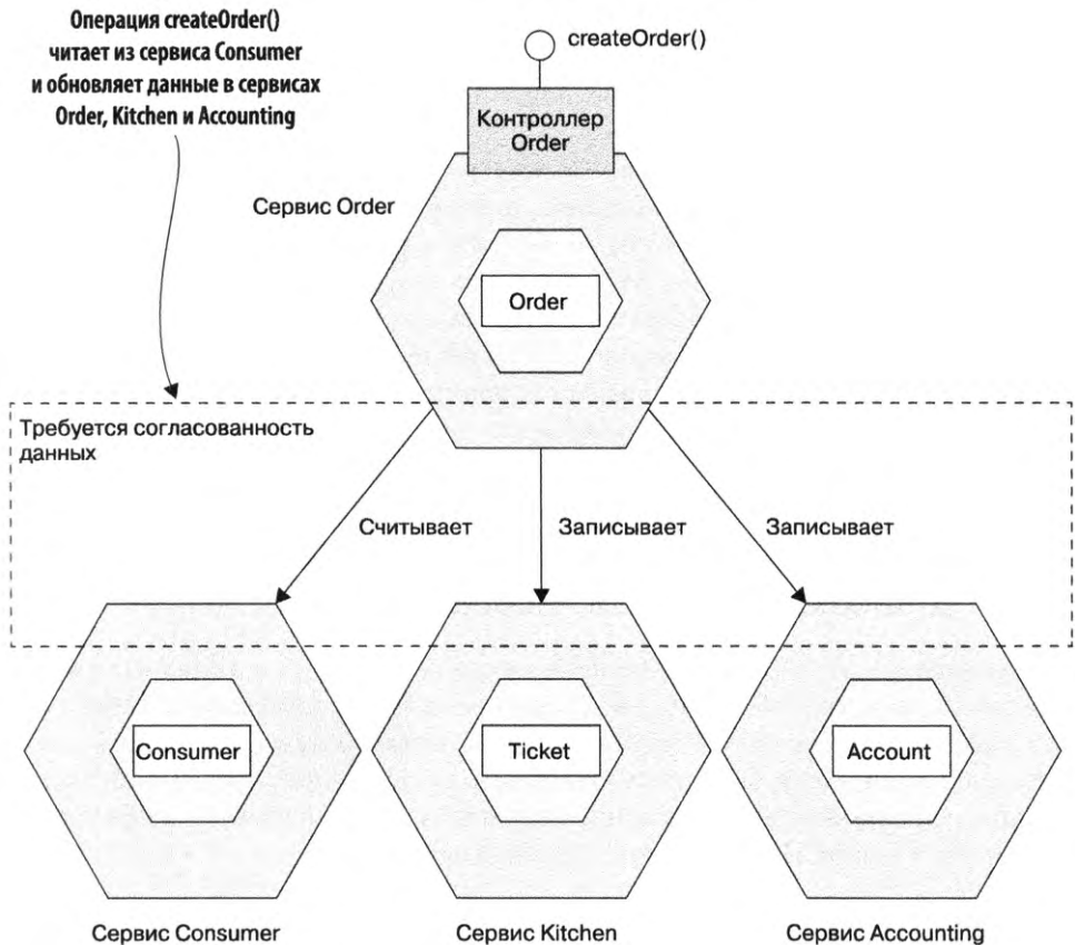
Рис. 4.1. Операция createOrder() обновляет данные в нескольких сервисах. Чтобы обеспечить согласованность между ними, она должна задействовать специальный механизм
