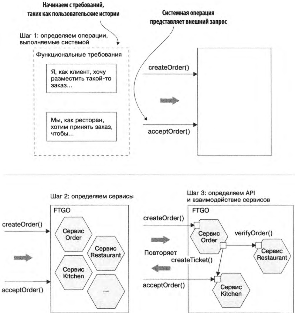
Рис. 2.5. Трехшаговый процесс описания микросервисной архитектуры приложения
