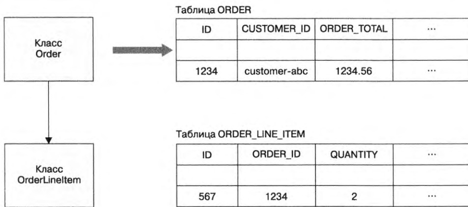
Рис. 6.1. Традиционный подход к сохранению информации подразумевает привязывание классов к таблицам, а объектов — к строкам в этих таблицах
