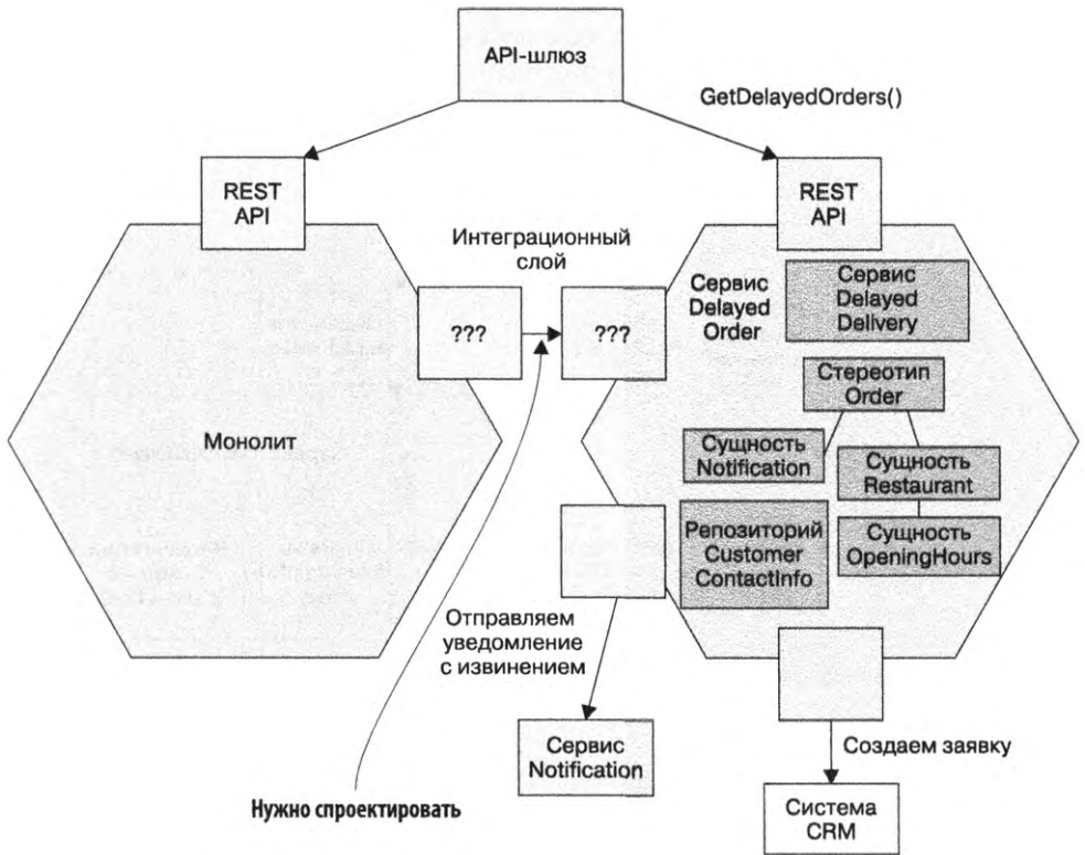
Рис. 13.14. Архитектура сервиса Delayed Delivery . Интеграционный слой предоставляет ему принадлежащие монолиту данные, такие как сущности Order и Restaurant , а также контактную информацию клиента
