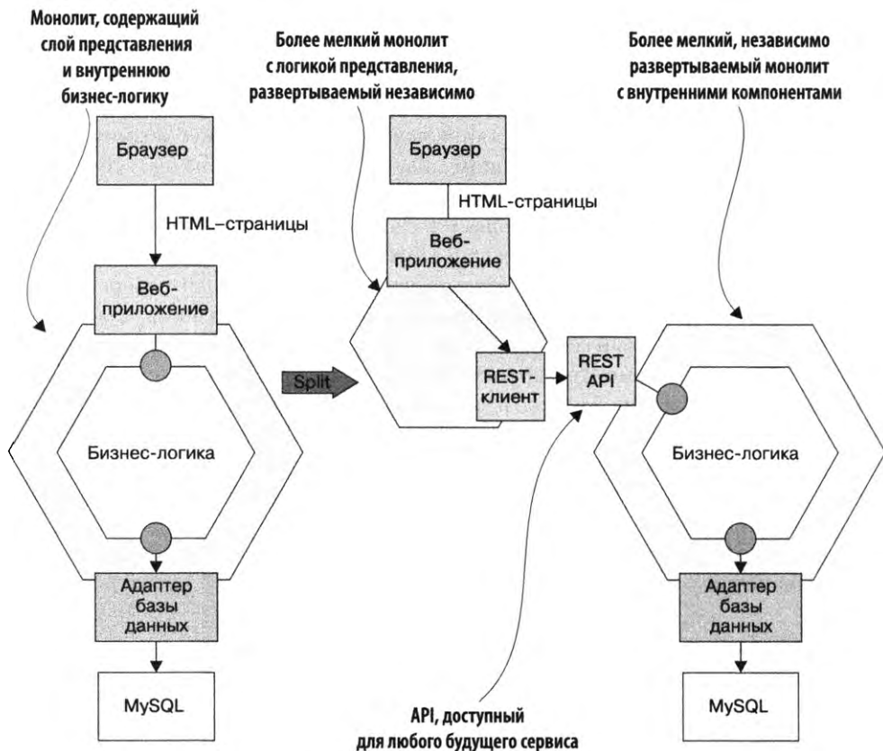
Рис. 13.3. Разделение клиентских и внутренних компонентов позволяет развертывать их отдельно друг от друга и открывает API для сервисов
