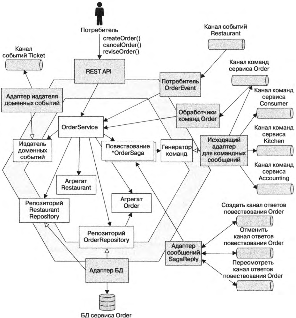
Рис. 5.12. Структура сервиса Order. Он имеет REST API для управления заказами и обменивается сообщениями и событиями с другими сервисами, используя несколько каналов сообщений
