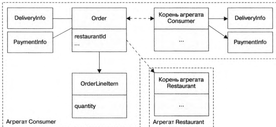
Рис. 5.8. Альтернативное решение описывает агрегат Consumer , который включает в себя классы Consumer и Order . Такой подход позволяет приложению атомарно обновлять заказчика и один или несколько его заказов
