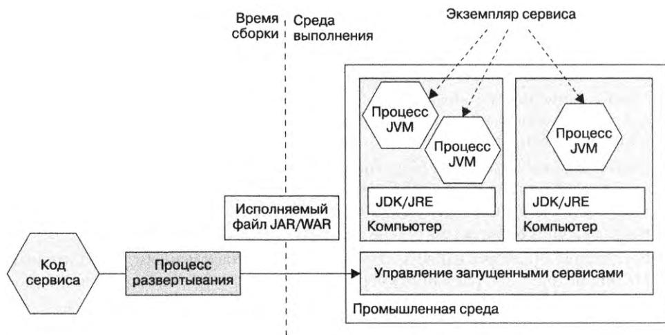
Рис. 12.3. Процесс развертывания собирает исполняемый JAR -файл и доставляет его в промышленную среду. В промышленной среде каждый экземпляр сервиса представлен JVM -машиной, запущенной на компьютере с установленным пакетом JDK или JRE
