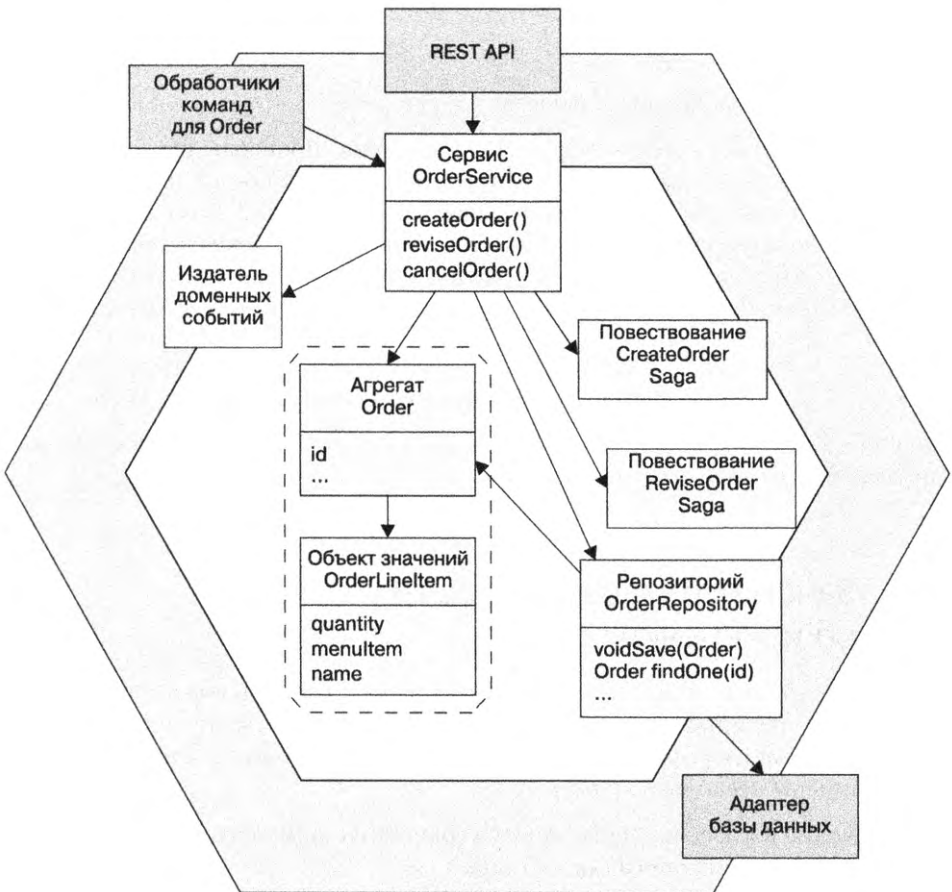
Рис. 5.9. Структура бизнес-логики сервиса Order на основе агрегатов
