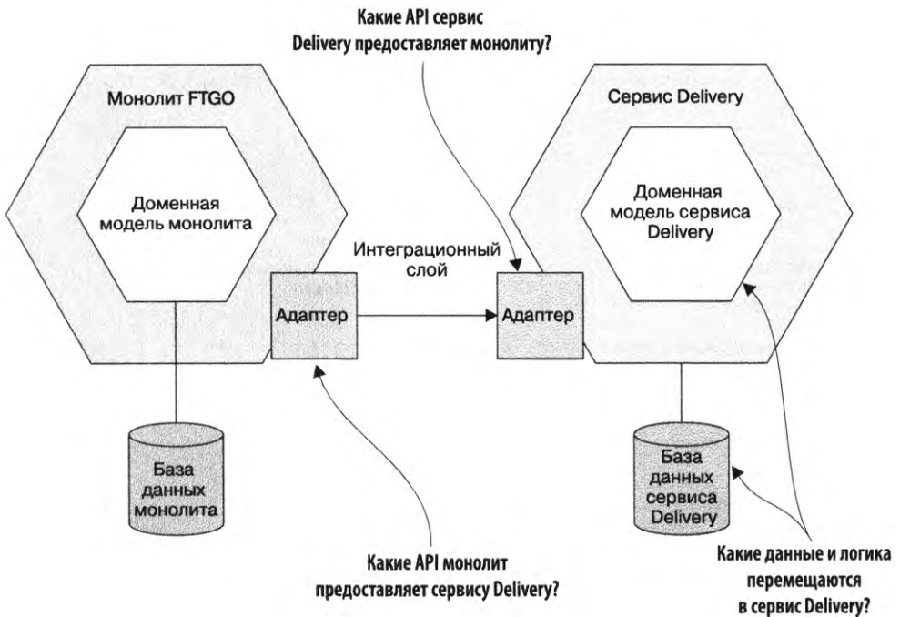
Рис. 13.17. Обобщенная схема приложения FTGO после извлечения сервиса Delivery. Монолит FTGO и сервис Delivery общаются с помощью интеграционного слоя, API которого размещены по обе стороны. Необходимо принять два ключевых решения: какие данные и функциональность перемещаются в сервис Delivery и через какие API монолит и сервис Delivery будут взаимодействовать между собой
