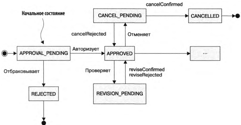
Рис. 5.14. Часть модели конечного автомата для агрегата Order
