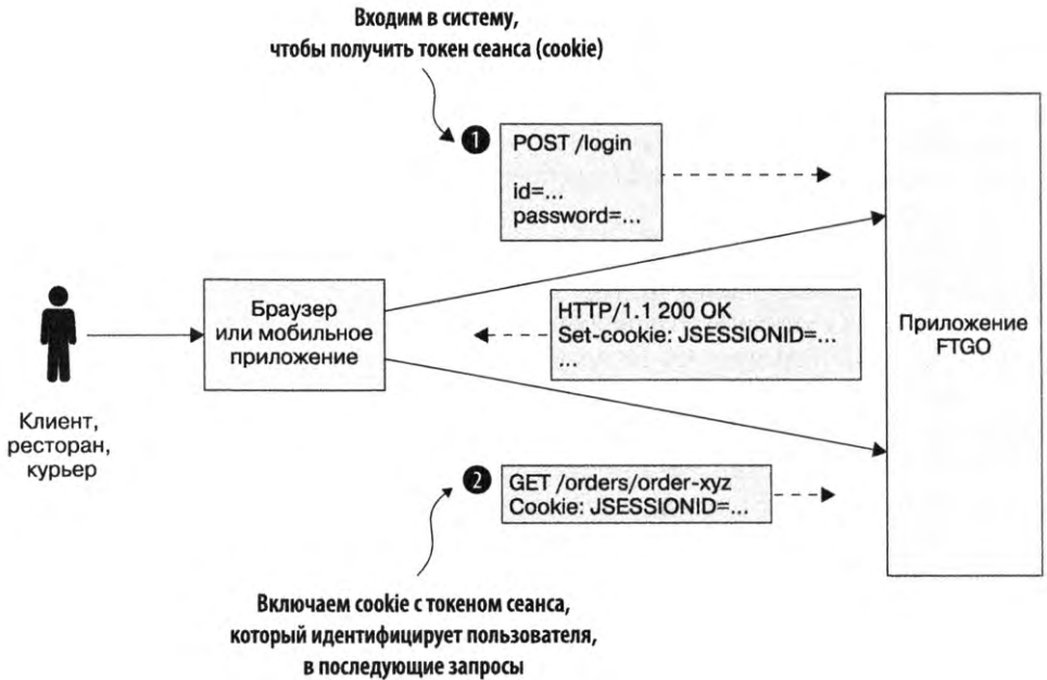
Рис. 11.1. Вначале клиент приложения FTGO входит в систему, чтобы получить токен сеанса, в качестве которого часто выступает cookie. Клиент включает этот токен в каждый последующий запрос, отправляемый приложению
