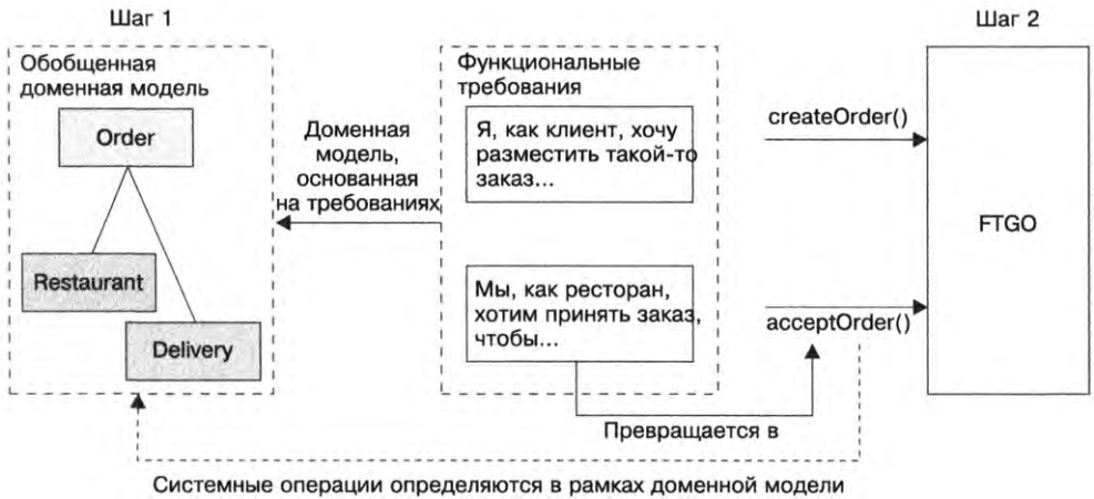
Рис. 2.6. Системные операции определяются на основе требований к приложению в ходе двухшагового процесса. На первом шаге создается обобщенная доменная модель. На втором шаге в рамках этой модели определяются системные операции
