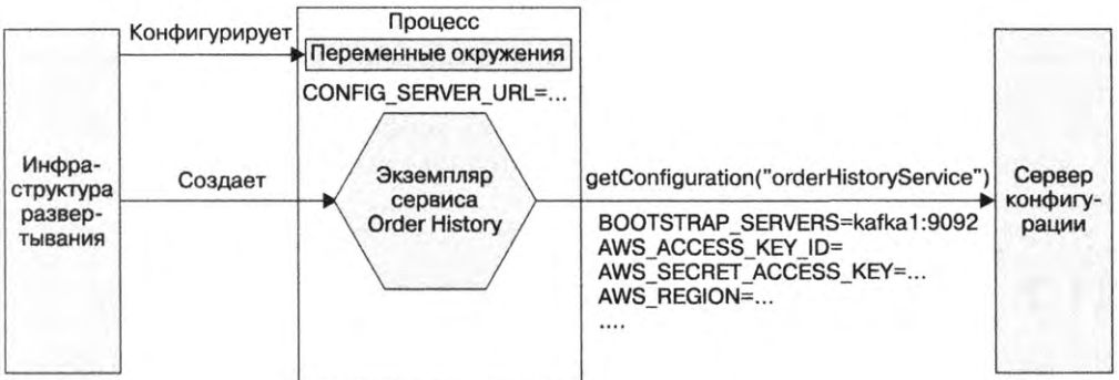
Рис. 11.8. При запуске экземпляр сервиса извлекает свои конфигурационные свойства из сервера конфигурации. Конфигурационные свойства для доступа к серверу конфигурации предоставляются инфраструктурой развертывания
